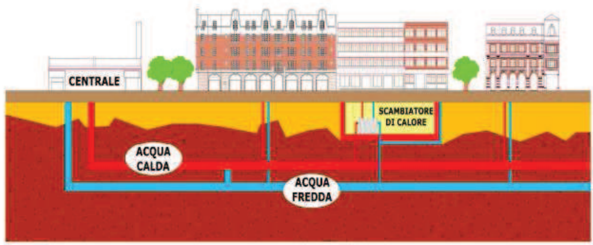
Figura 1: Schema per un impianto di teleriscaldamento
